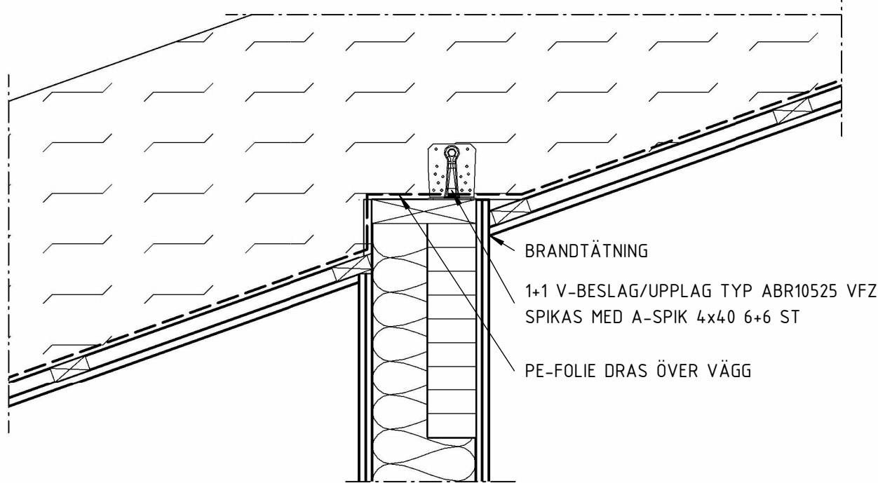
03 1 : 10 TAKSTOL PÅ FLÄKTRUMSVÄGG
