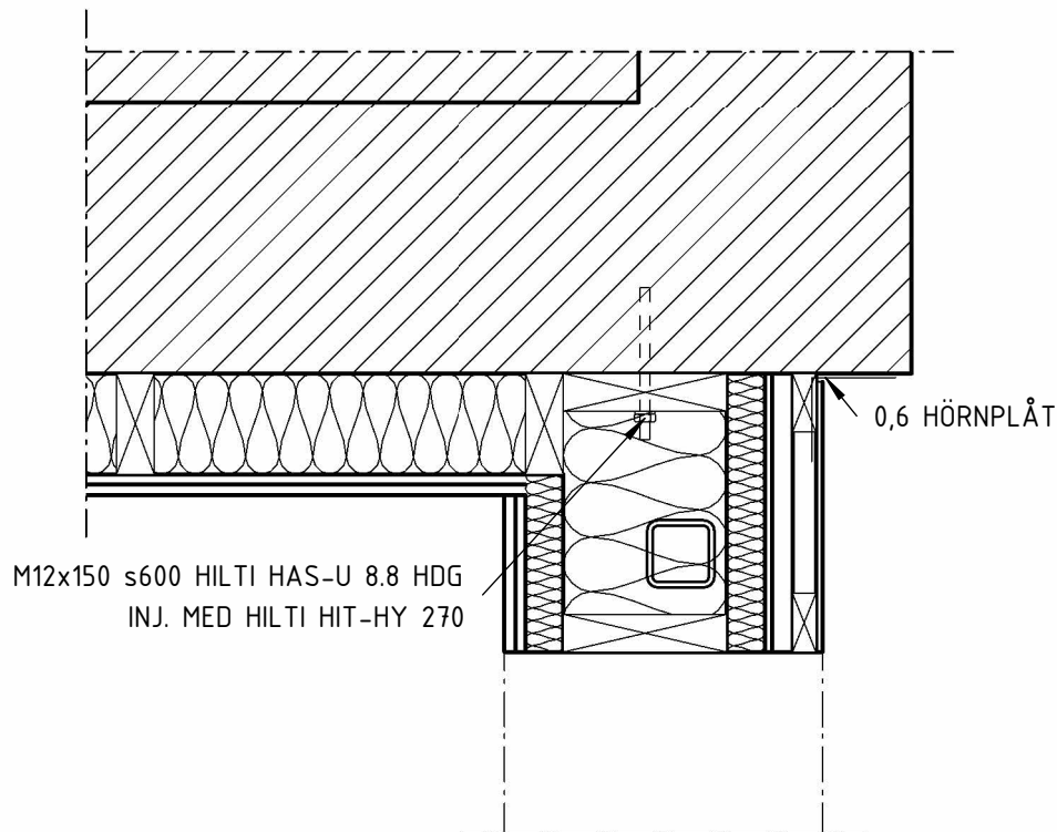
09 1 : 10 ANSLUTNING MOT BEFINTLIGT
