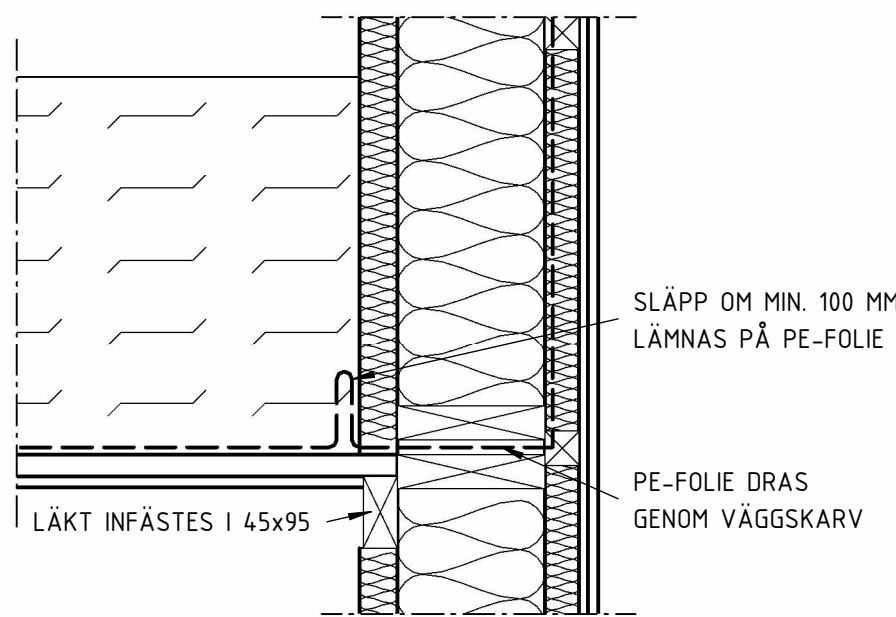
06 1 : 10 ÖVERGÅNG TAKSTOLSTYPER
