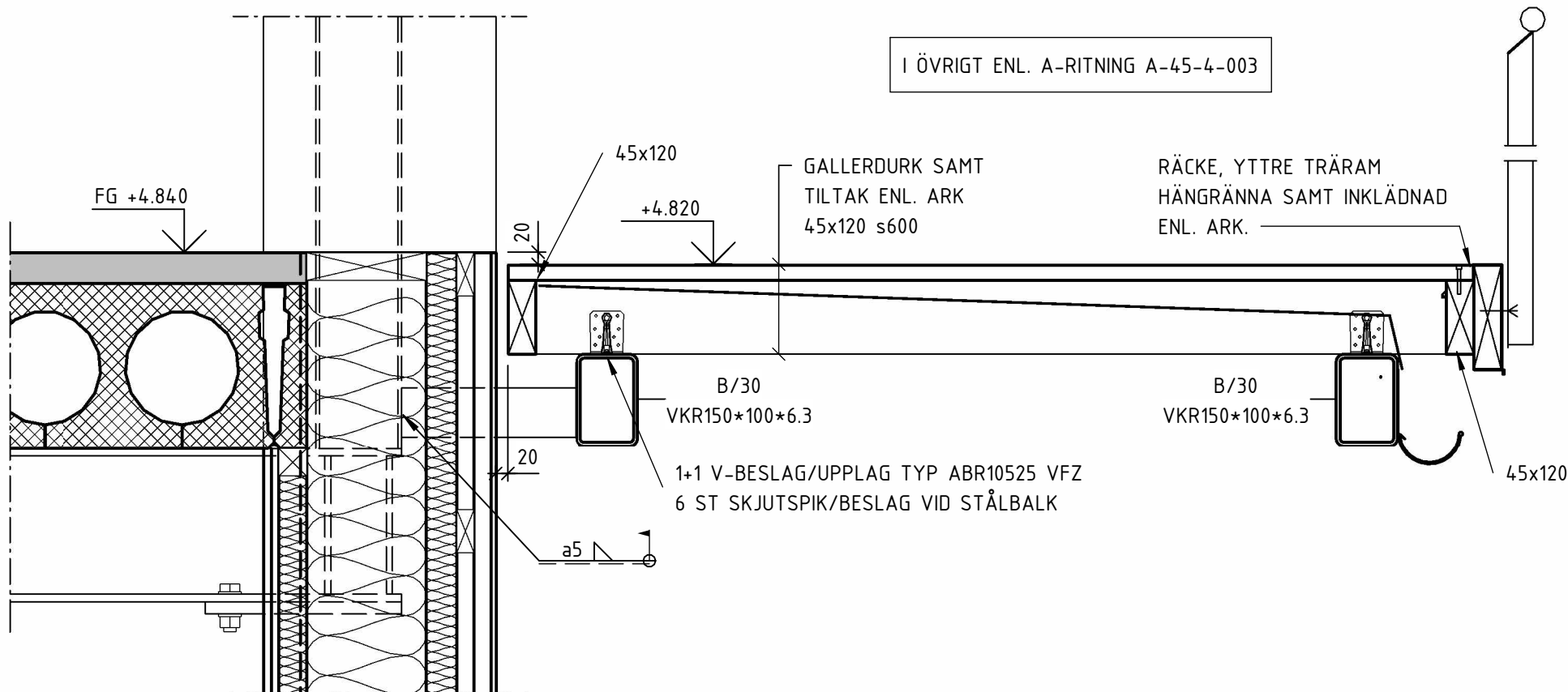
07 1 : 10 FLÄKTRUMSBALKONG TVÄR
