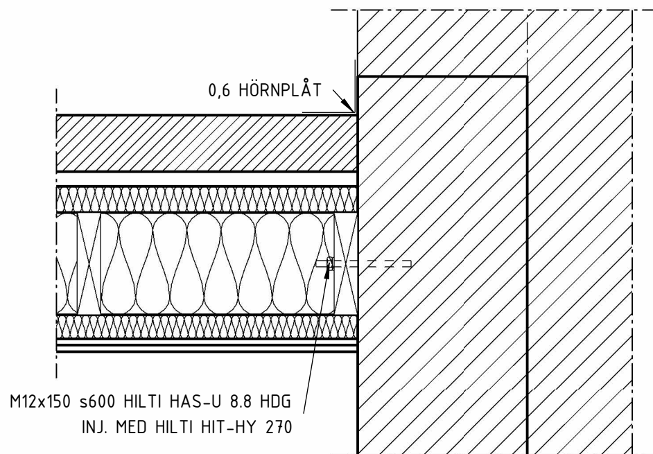
10 1 : 10 ANSLUTNING MOT BEFINTLIGT
