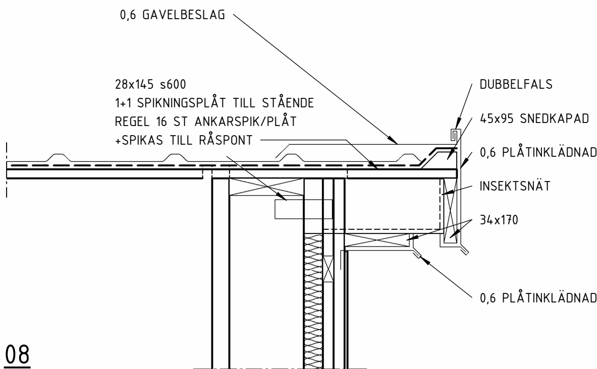
08 1 : 10 GAVEL
