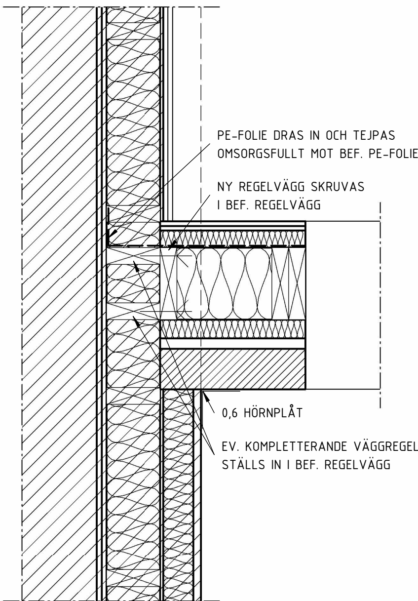
11 1 : 10 ANSLUTNING MOT BEFINTLIGT
