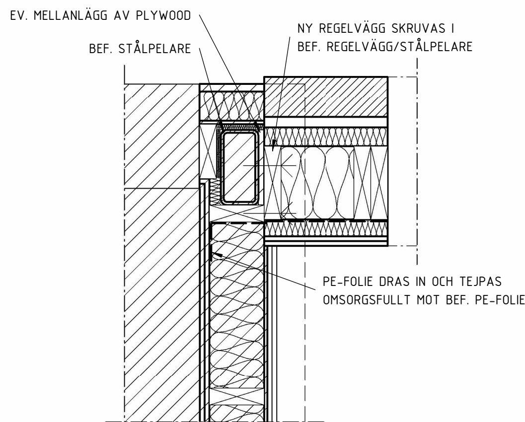
12 1 : 10 ANSLUTNING MOT BEFINTLIGT
