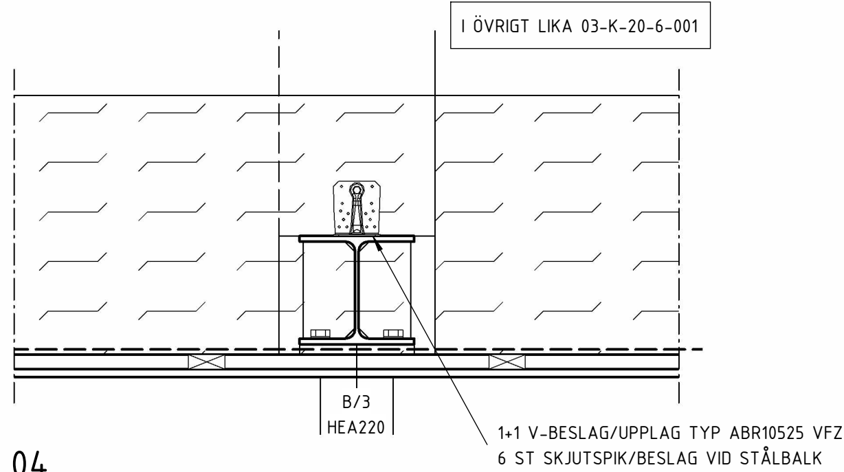
04 1 : 10 TAKSTOL PÅ STÅLBALK
