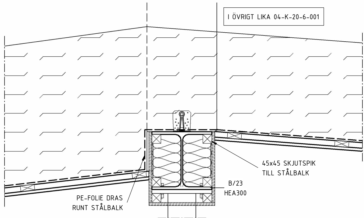
05 1 : 10 TAKSTOL PÅ STÅLBALK
